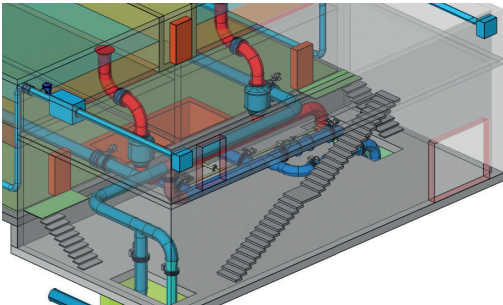
HB Birkenfeld Techn. Ausrüstung – 3 D-Modell
